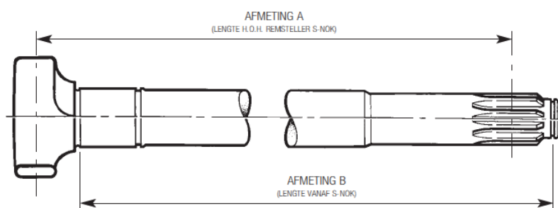
Remsleutel Type 'A' – gerolde vertanding – met gestante remankerplaat (vanaf April 2001)
