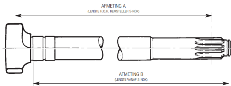
Remsleutel Type 'Z' – gerolde vertanding – met gestante remankerplaat
